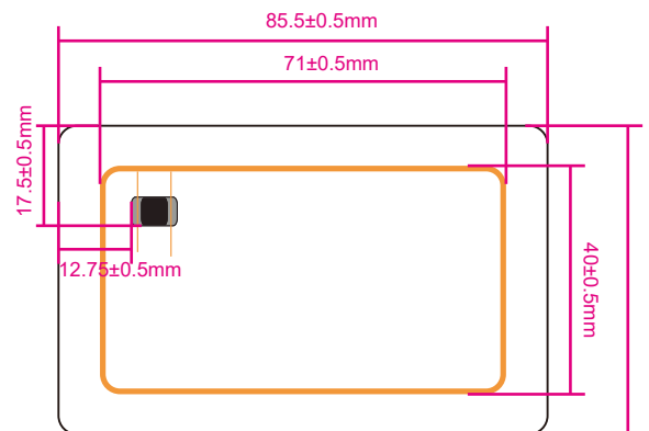
天线 (Antenna)
